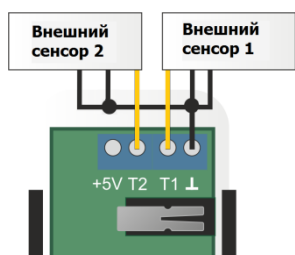
Рисунок 8.1 – Схема подключения внешних сенсоров DS18B20
