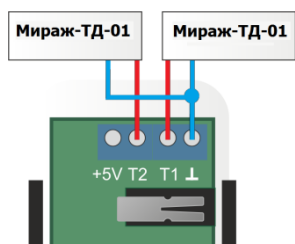
Рисунок 8.2 – Схема подключения внешних сенсоров Мираж-ТД-01
