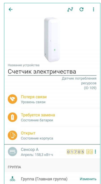
Рисунок 12.3 – Экран настройки датчика (батарея разряжена, корпус вскрыт, потеря связи)
