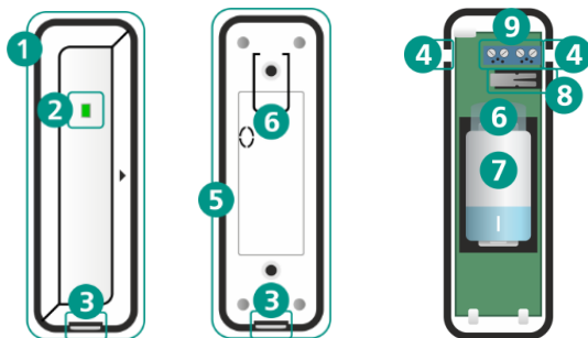
Рисунок 2.1 – Внешний вид датчика
